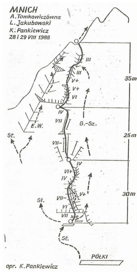
Fot. 48. Schemat topograficzny nowej drogi wspinaczkowej „2+1” na Mniechu Źródło: „Taternik” 1988, nr 2, s. 69.
